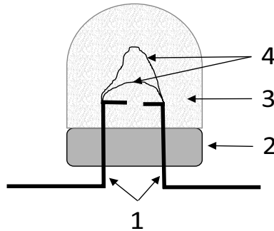
Rys. 5. Schemat zapłonika elektrycznego: 1 – ołowiane przewody; 2 – podstawka główki zapalczącej; 3 – mieszanina pirotechniczna; 4 – cienkie druty oporowe
